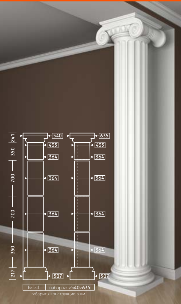
СТВОЛ 4.12.003
