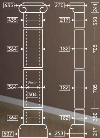
СТВОЛ 4.16.005
