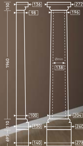
БАЗА 1.17.600
