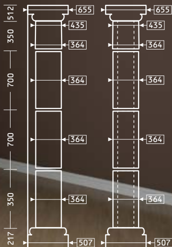
СТВОЛ 4.12.005
