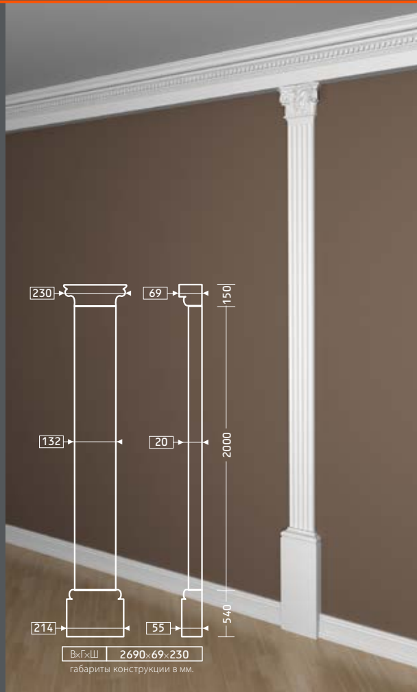
КАПИТЕЛЬ 1.21.001 СТВОЛ 1.22.010
