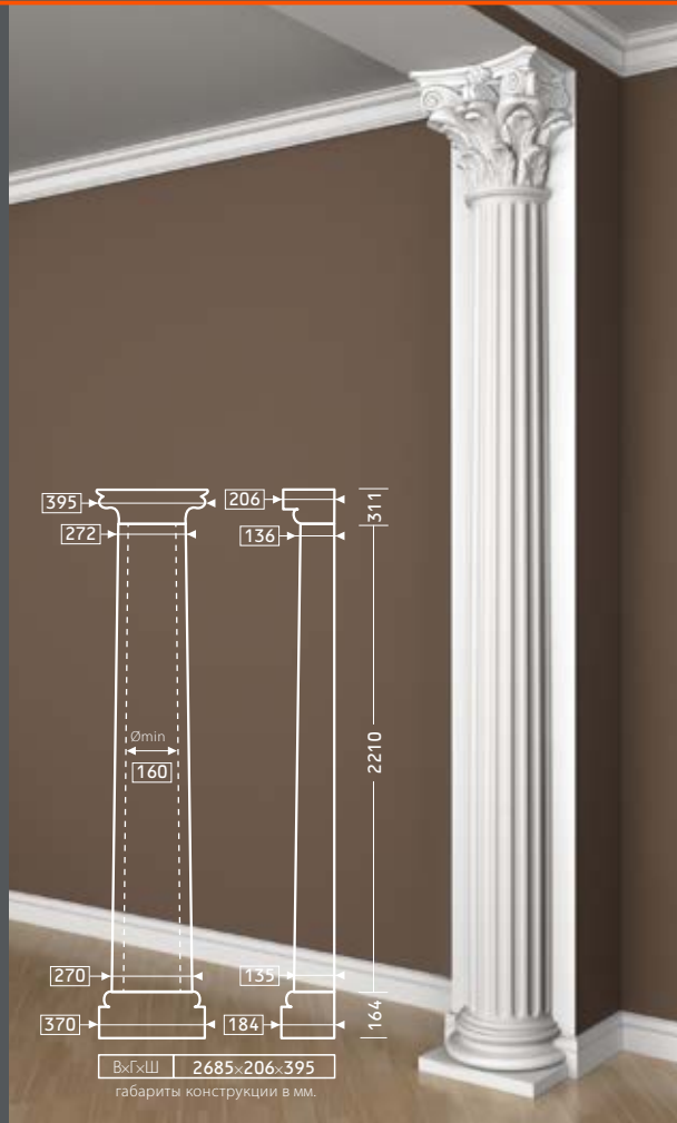
КАПИТЕЛЬ 4.15.301 СТВОЛ 4.16.301
