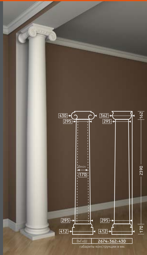
КАПИТЕЛЬ 4.11.201 СТВОЛ 4.12.202
