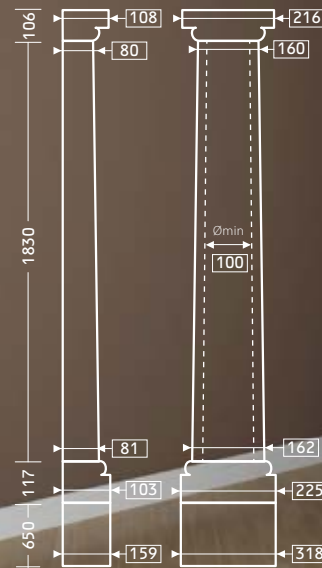
БАЗА 1.17.700
