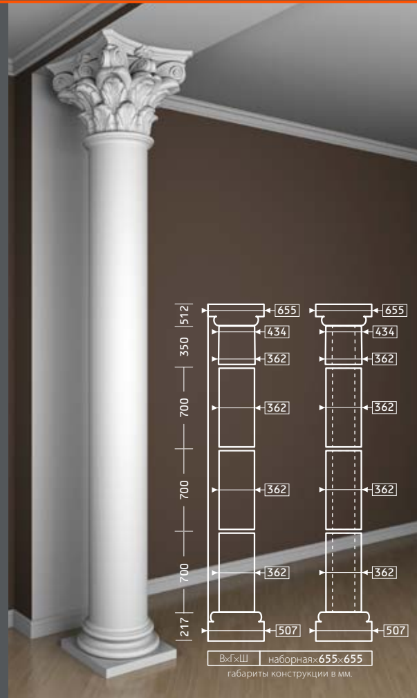
КАПИТЕЛЬ 4.11.302
