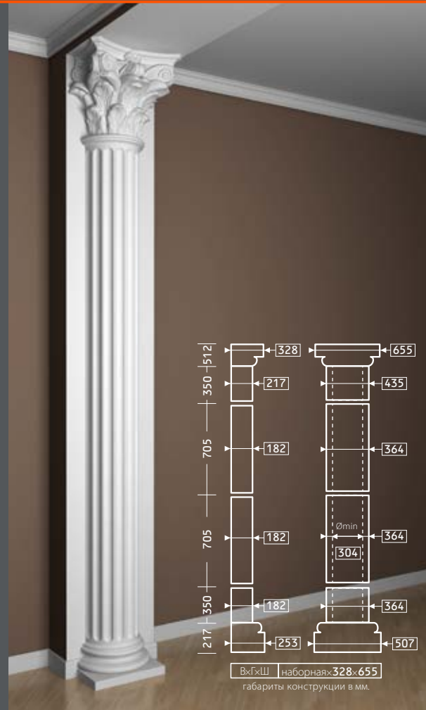
КАПИТЕЛЬ 4.15.302 СТВОЛ 4.16.003
