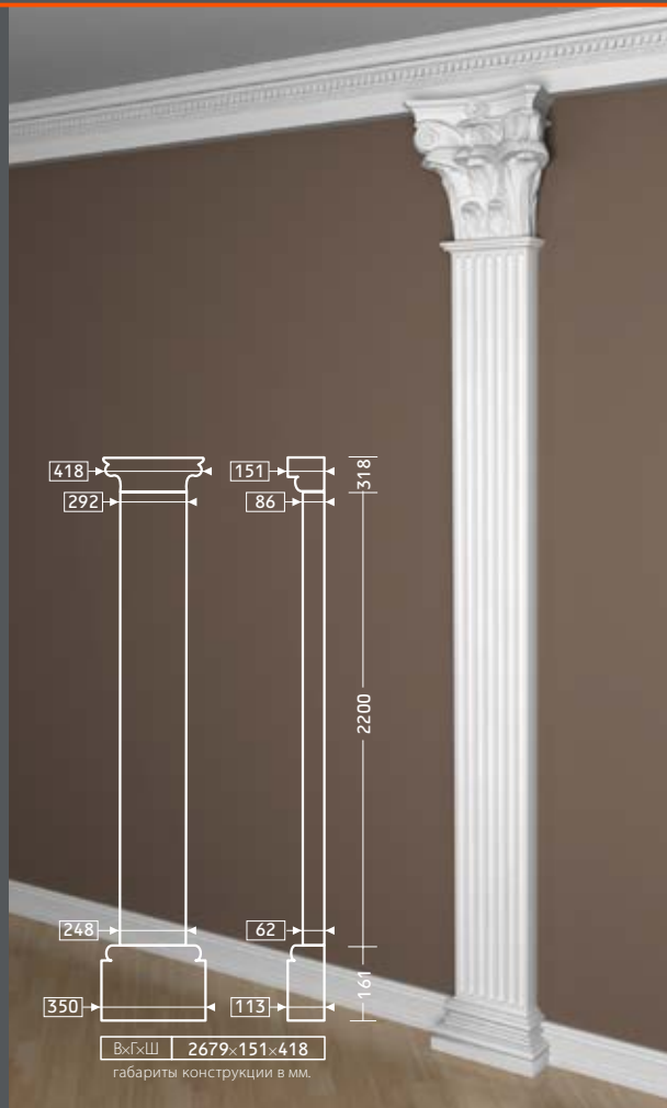
КАПИТЕЛЬ 4.21.301 СТВОЛ 4.22.301
