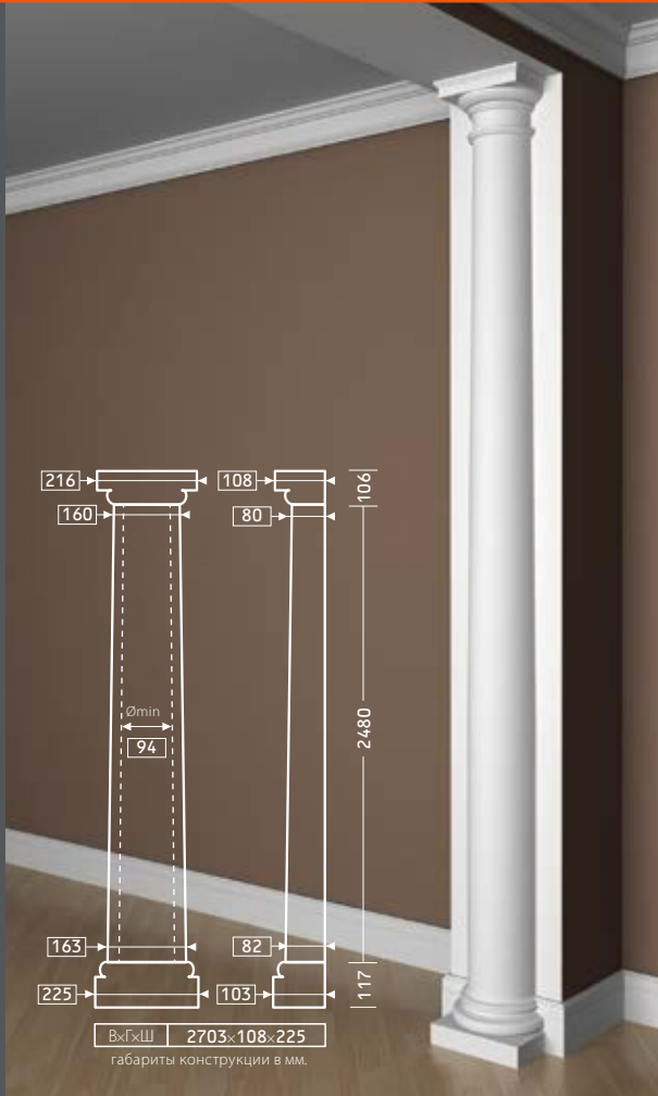
КАПИТЕЛЬ 1.15.008 СТВОЛ 1.16.061
