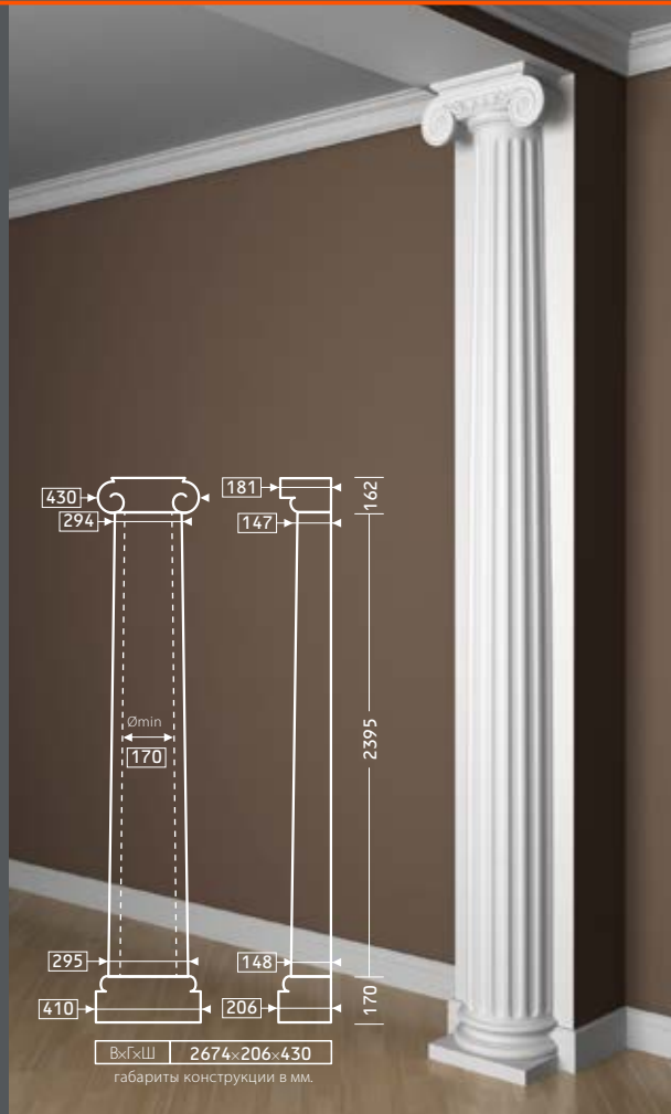
КАПИТЕЛЬ 4.15.201 СТВОЛ 4.16.201
