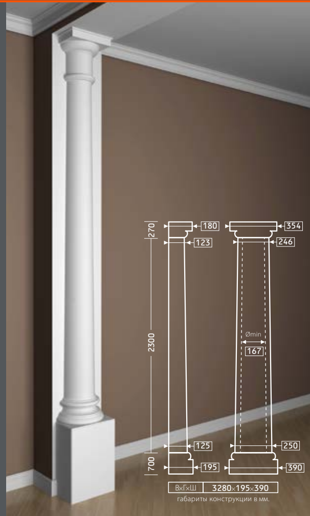
КАПИТЕЛЬ 1.15.002 СТВОЛ 1.16.020
