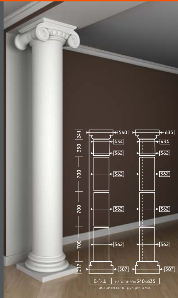
КАПИТЕЛЬ 4.11.202
