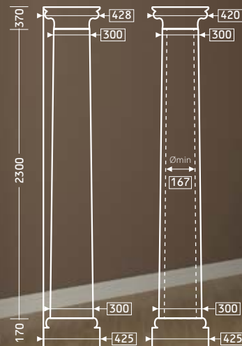
БАЗА 1.13.400
