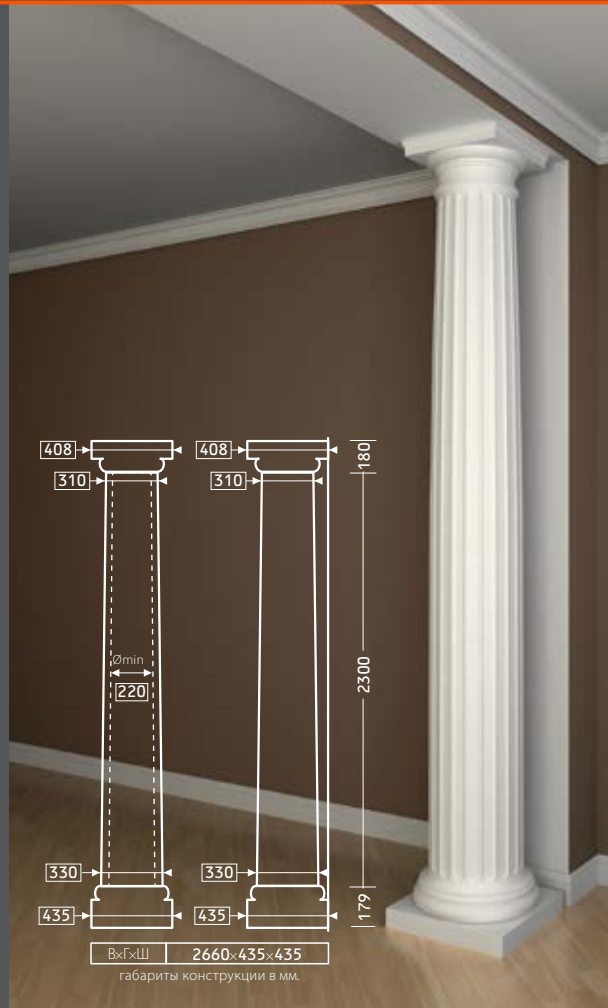
КАПИТЕЛЬ 4.11.101 СТВОЛ 4.12.102
