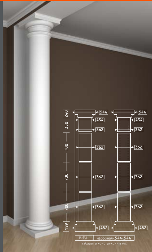
КАПИТЕЛЬ 4.11.102 СТВОЛ 4.12.001
