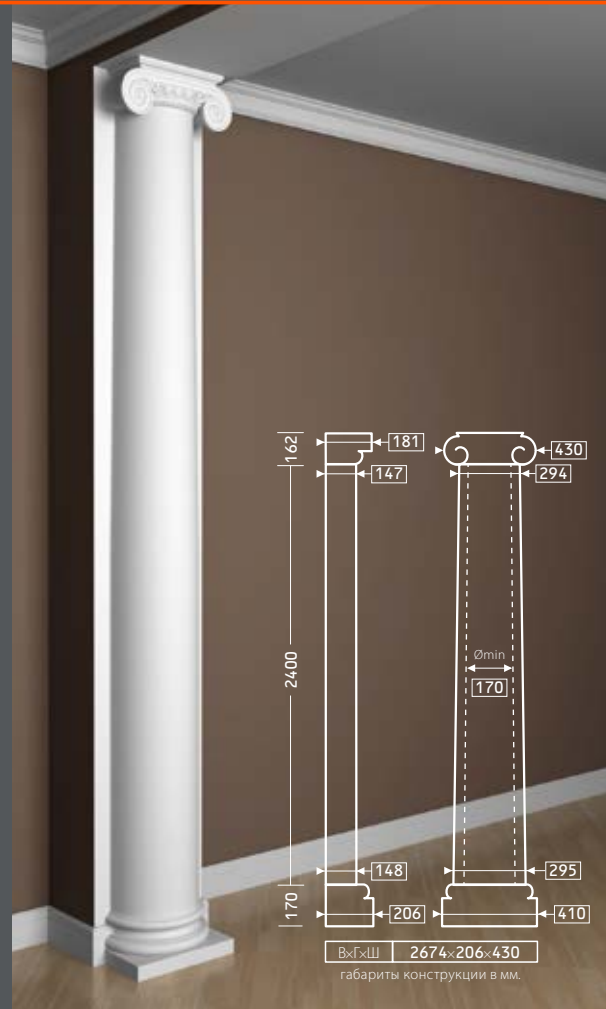
КАПИТЕЛЬ 4.15.201 СТВОЛ 4.16.202
