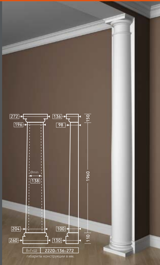
КАПИТЕЛЬ 1.15.005 СТВОЛ 1.16.050
