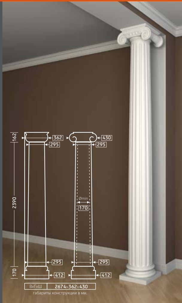
КАПИТЕЛЬ 4.11.201 СТВОЛ 4.12.201
