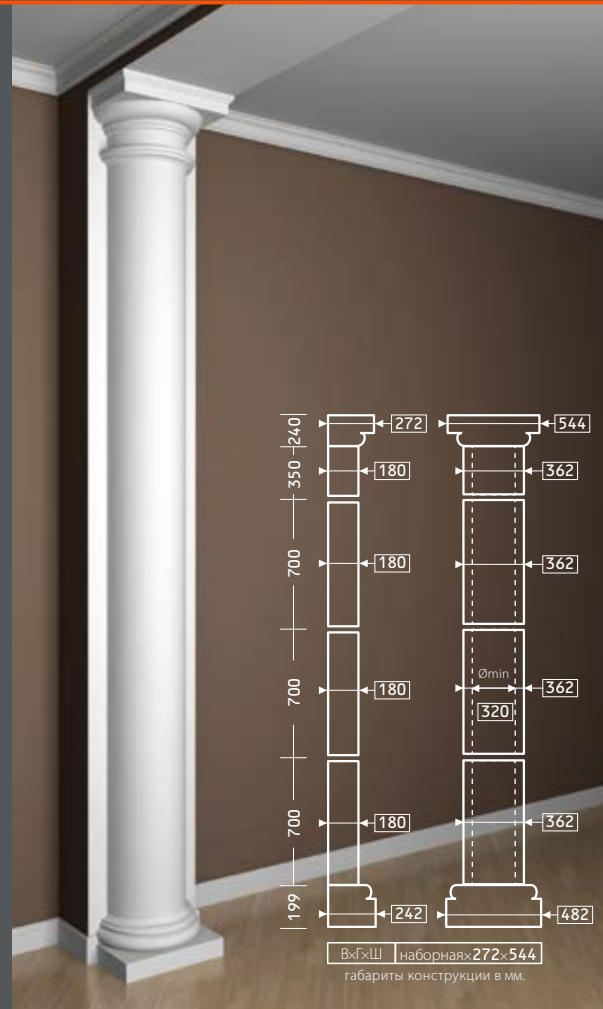
КАПИТЕЛЬ 4.15.102 СТВОЛ 4.16.001
