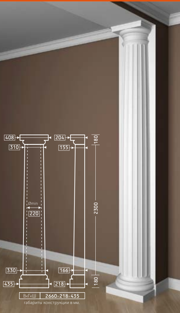
КАПИТЕЛЬ 4.15.101 СТВОЛ 4.16.102
