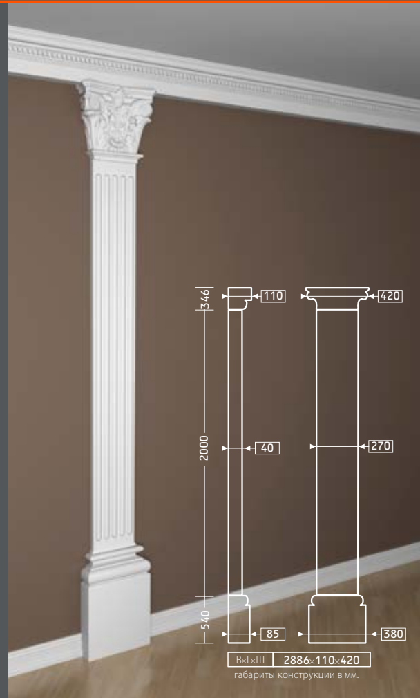
КАПИТЕЛЬ 1.21.002 СТВОЛ 1.22.020
