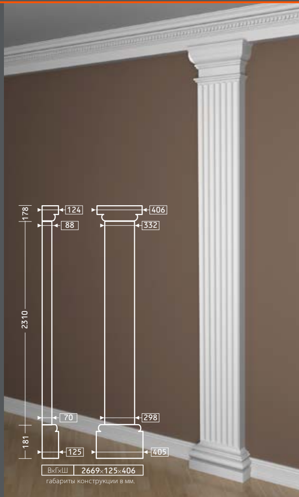
КАПИТЕЛЬ 4.21.101 СТВОЛ 4.22.101
